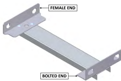
'STARTER'
